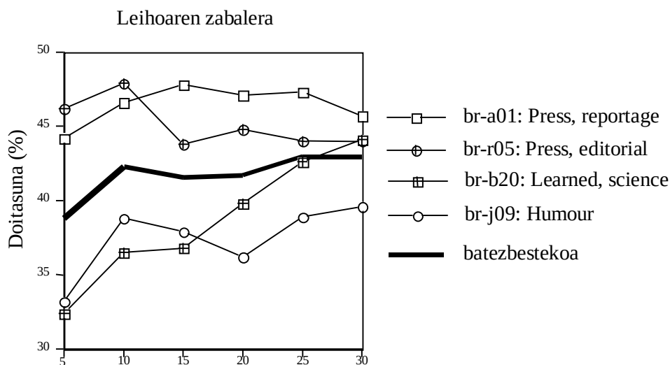
21. irudia: testuinguruaren zabalaren eragina testu fitxategietan
