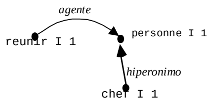
24. irudia: reunir-en hautapen-murritzpena chef-ek nola bete dezakeen
