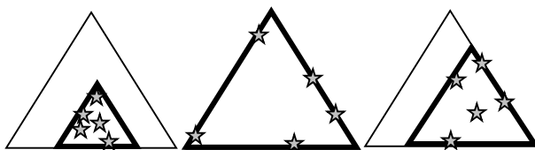
2. irudia: arrasto multzoak estaltzen dituzten azpizuhaitz minimoak (marra lodiagoak).
