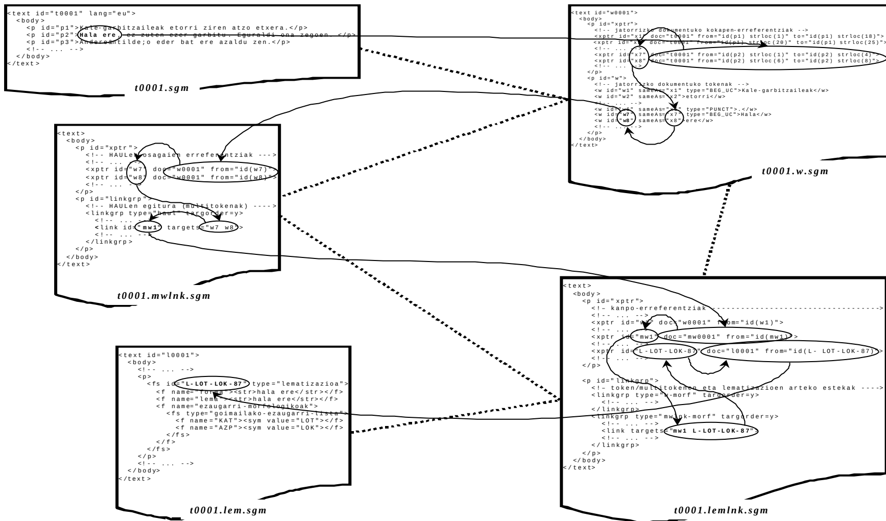
II.4 irudia.- Lematizatzailearen irteera: dokumentu-amaraunaren adibide bat.
