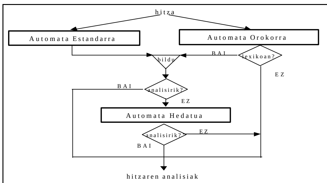
III.5 irudia.- Analizatzaile inkrementalaren funtzionamendua.
