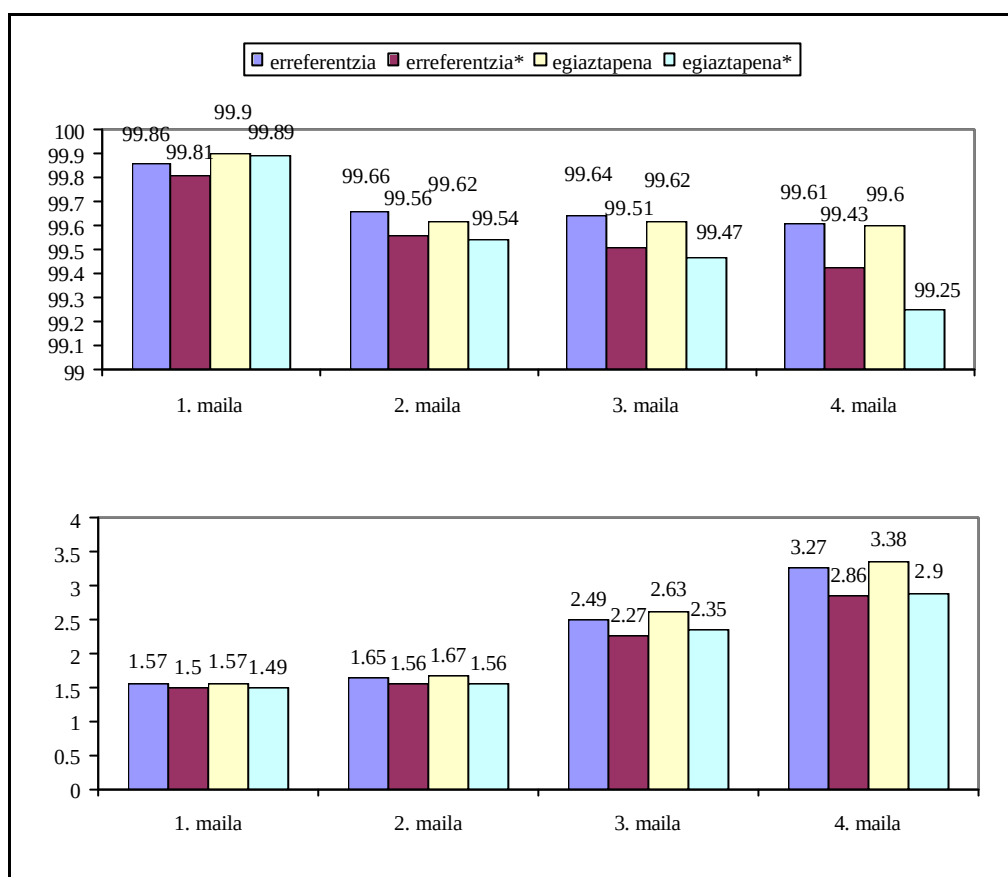
IV.1 irudia.- Zuzentasuna eta analisi kopurua etiketa-mailaren arabera.
