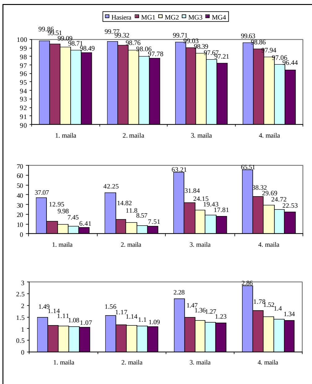
C.1 irudia.- MGren emaitzak etiketatze-mailaren arabera erreferentzia-corpusean.
