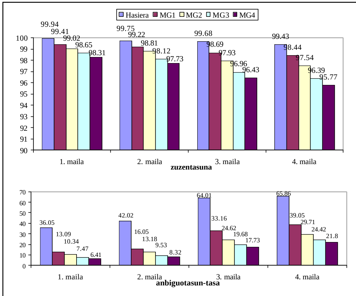
VI.1 irudia.- MG aplikatu aurretik eta ondorengo emaitzak etiketatze-mailaren arabera.
