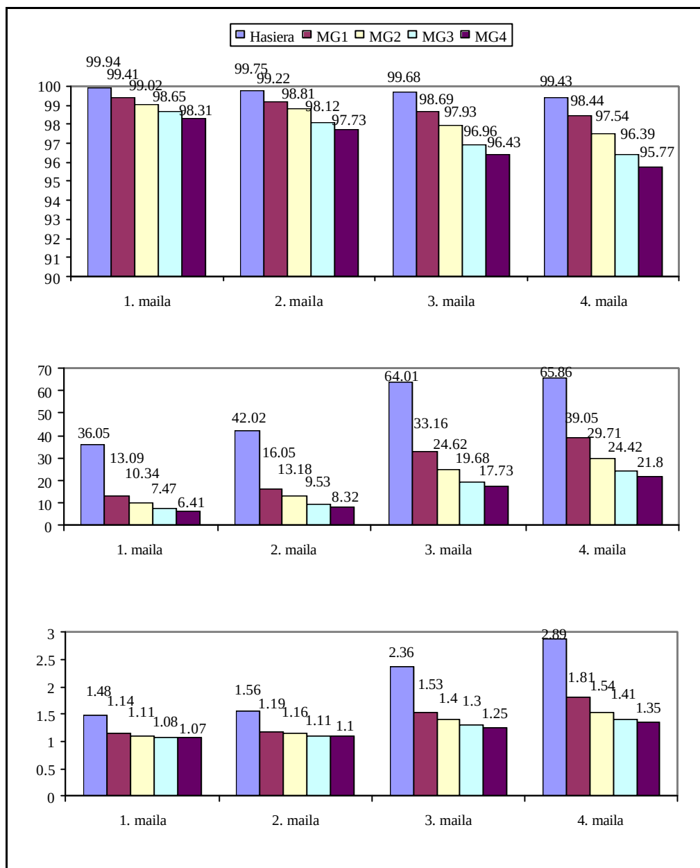
C.2 irudia.- MGren emaitzak etiketatze-mailaren arabera egiaztapen-corpusean.
