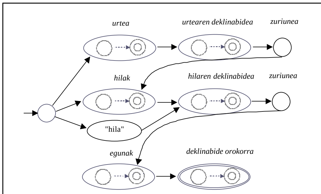
V.3 irudia. - Daten ezagutzailearen lexikoien antolakuntza.
