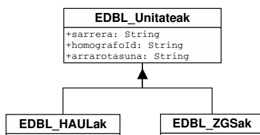
IV.11 Irudia: EDBL datu-basearen BEKa: Hitz Anitzeko Unitate Lexikalak (HAUL) eta Zuriunerik Gabeko Sarrerak (ZGS).
