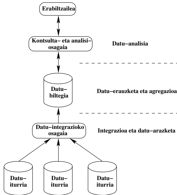
III.2 Irudia: Datu-biltegi sistema baten oinarriko arkitektura
