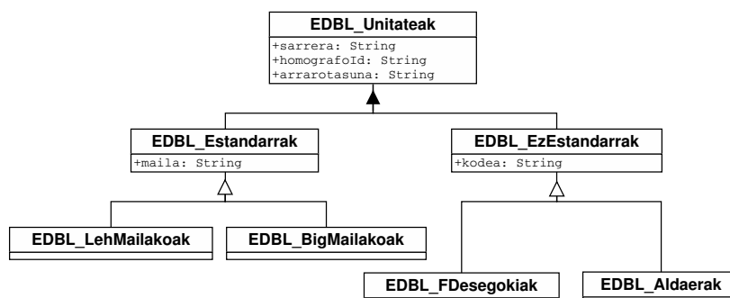
IV.10 Irudia: EDBL datu-basearen BEKa: unitate estandar eta ez-estandar- rrak.
